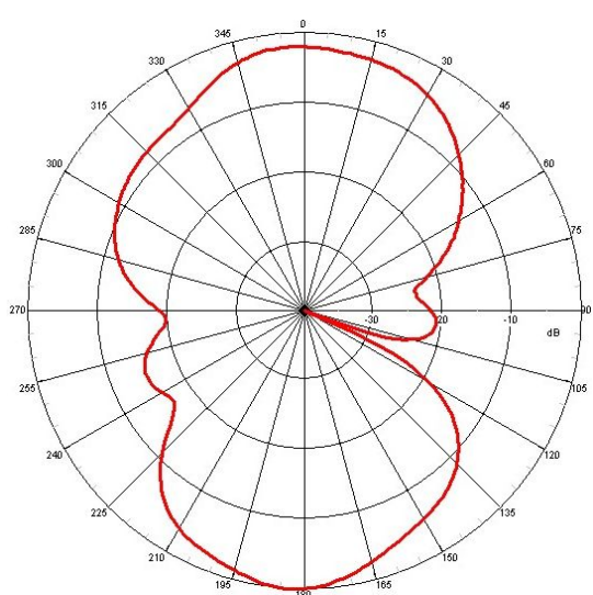
E-PLANE
