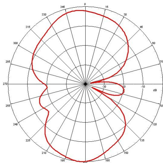
E-PLANE
