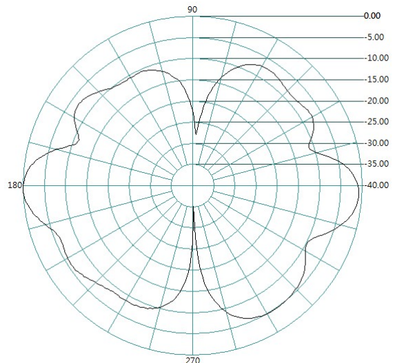
E-PLANE
